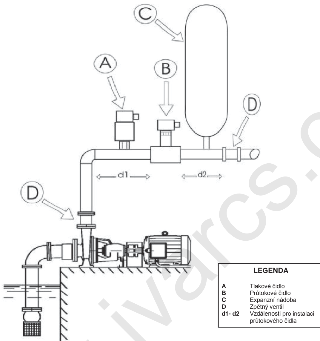
Obrázek 5: Hydraulická instalace
