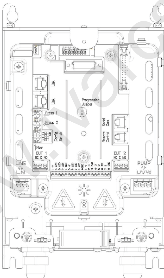
Obrázek 4: Elektrické zapojení
